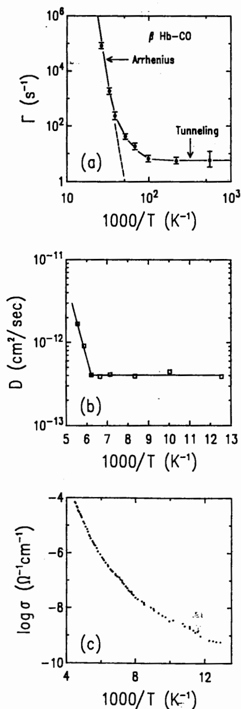
Fig. 1: Tieftemperatur - Reaktionsraten von drei verschiedenen Prozessen, bei denen der Tunnel-effekt die Rate entscheidend mitbestimmt. (a) Reaktionsrate \Gamma für die Bindung von Kohlenmonoxid an Eisen im Hämoglobin. (b) Wasserstoffdiffusion D auf der Oberfläche von Wolfram. (c) Elektrische Leitfähigkeit einer Titan-Vanadium-Legierung.
