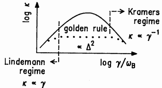
Fig. 3: Qualitative Abhängigkeit der diffusiven Transmission \kappa (d. h. Wert des Raten-Vorfaktors) bei thermischer Aktivierung als Funktion der Dämpfung \gamma . Die entsprechenden stochastischen Teilchentrajektorien an der Barrierschwelle eines symmetrischen Doppeltopfes sind in Figur (i) - (iii) aufgezeichnet. (i) Relaxationsverlauf bei kleiner Dämpfung (Energie Diffusion); (ii) überdämpfte Relaxation bei großer Dämpfung; (iii) Teilchenbewegung bei frequenzabhängiger Dämpfung.
