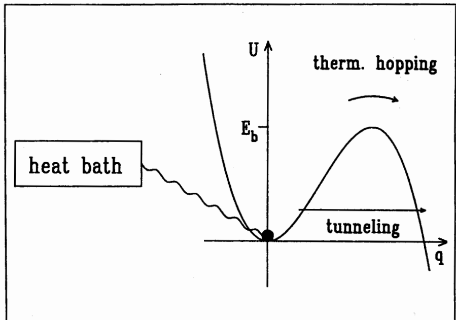
Fig. 2: Der Metastabile Zustand. Das Teilchen kann aufgrund thermischer Aktivierung über den Potentialberg hüpfen oder aber mittels Tunneleffekts durchqueren.
