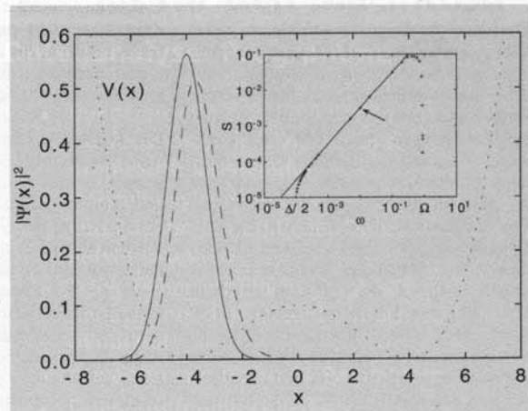
Abb. 2: Kohärente Unterdrückung des Tunnelns in einem symmetrischen Doppelmuldenpotential mit periodischem Antrieb (gepunktet, Gl. 1 mit D = 2 bei t = \pi/2\omega , Ordinate in willkürlichen Einheiten) an einer Überkreuzung der dem Grundzustandsdublett entsprechenden Quasienergien. Die gestrichelte Kurve zeigt die maximale Verschiebung eines in der linken Mulde präparierten Wellenpakets (durchgezogen) im Laufe seiner Zeitentwicklung. Die Wahrscheinlichkeit, im Ausgangszustand zu verbleiben, ist im Rahmen einer Zweiniveuaunäherung durch den Ausdruck P(t) \sim \cos^2[J_0(S\mu/\hbar\omega)\Delta t/2\hbar] gegeben, in dem \mu das Übergangsdipolmoment bezeichnet. Die Nullstellen der nullten Bessel-Funktion J_0(S\mu/\hbar\omega) bestimmen approximativ die Lage der Kreuzungen in der (\omega, S) -Ebene. In der Einfügung wird diese Mannigfaltigkeit (durchgezogen) mit Punkten der entsprechenden exakten Kurve (Kreuze) verglichen. Der Pfeil markiert die für das Hauptbild gewählten Parameterwerte.
