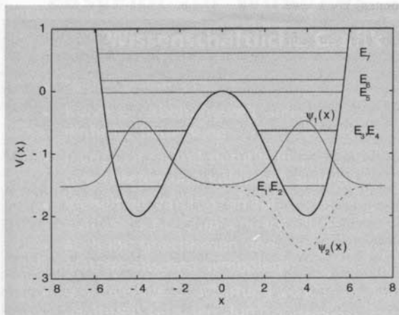
Abb. 1: Kohärentes Tunneln in einem symmetrischen Doppelmuldenpotential ohne Antrieb (dicke Linie, nach Gl. 1 mit D = 2 und S = 0 ). Die Aufspaltung der untersten beiden Tunnel-dubletts im Energiespektrum (horizontale Linien) wird im Druck nicht mehr ( E_1, E_2 ) bzw. gerade noch ( E_3, E_4 ) aufgelöst. Der Grundzustand \psi_1(x) (durchgezogen, Ordinate in willkürlichen Einheiten) ist von gerader Parität, der erste angeregte Zustand \psi_2(x) (gestrichelt) von ungerader Parität. Für einen in der linken Mulde konzentrierten Anfangszustand |\psi_{\text{links}}\rangle = (|\psi_1\rangle + |\psi_2\rangle)/\sqrt{2} lautet die Wahrscheinlichkeit, in diesem Zustand zu bleiben, P(t) = \cos^2(\Delta t/2\hbar) , wo \Delta = E_2 - E_1 die Aufspaltung des untersten Dubletts angibt.
